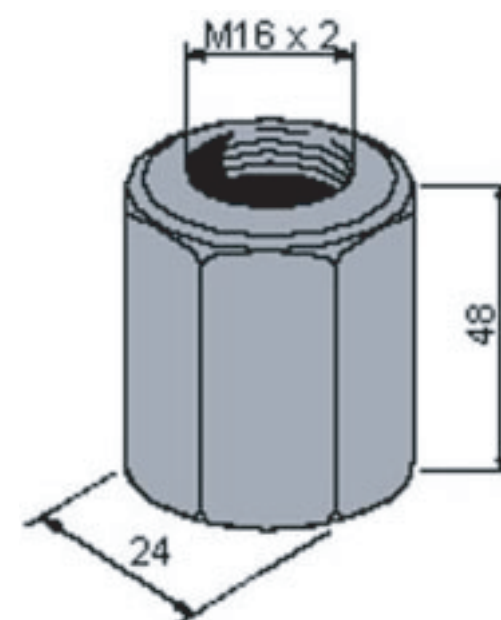
MODELO: M16 x 3D ARTICULO 603 - DIN 6330 B
