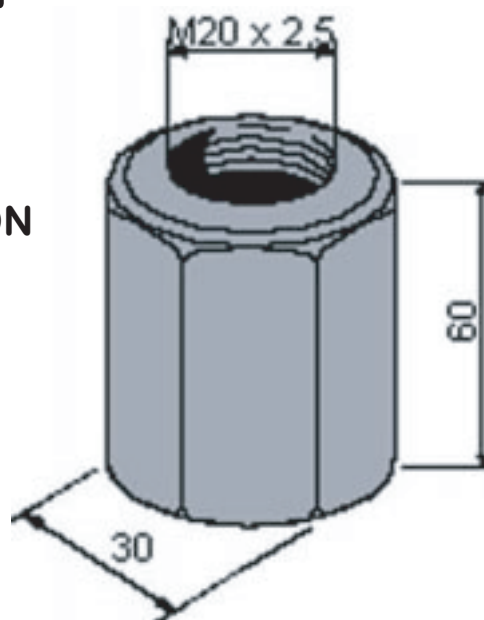
MODELO: M20 x 3D ARTICULO 603 - DIN 6330 B
