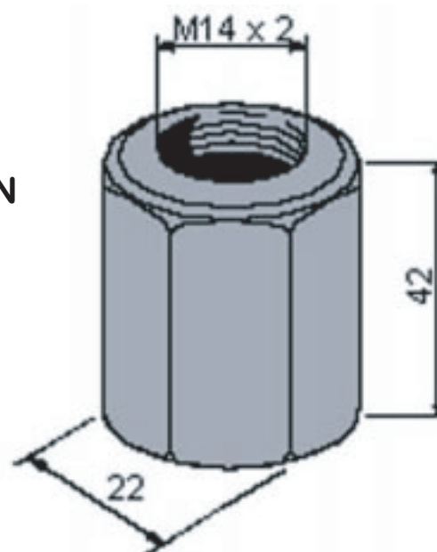
MODELO: M14 x 3D ARTICULO 603 - DIN 6330 B
