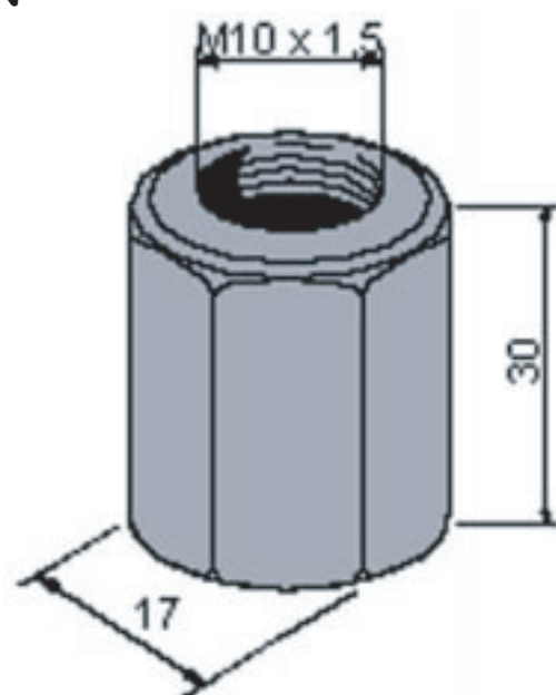
MODELO: M10 x 3D ARTICULO 603 - DIN 6330 B
