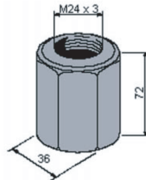
MODELO: M24 x 3D ARTICULO 603 - DIN 6330 B
