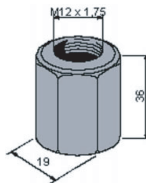
MODELO: M12 x 3D ARTICULO 603 - DIN 6330 B
